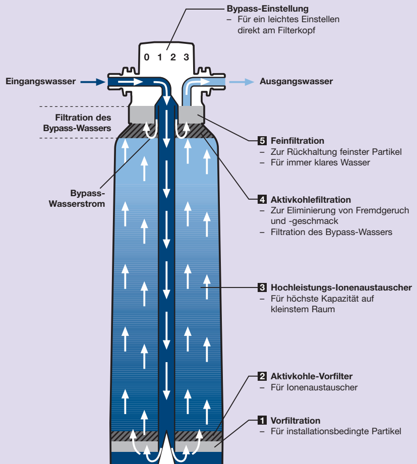
Aufbau einer BWT bestprotect Filterkerze mit 5-fach-Filtration
